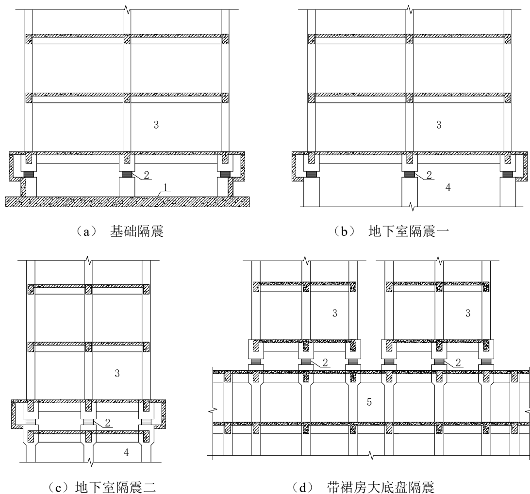
图 7.2.1 隔震层布置示意图
