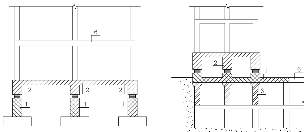
(a) 无地下室隔震建筑
