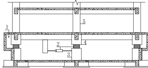
图 2.1.2 隔震结构各部分示意图
