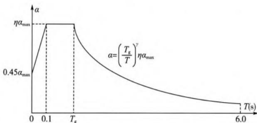
图 4.2.1 地震影响系数曲线
