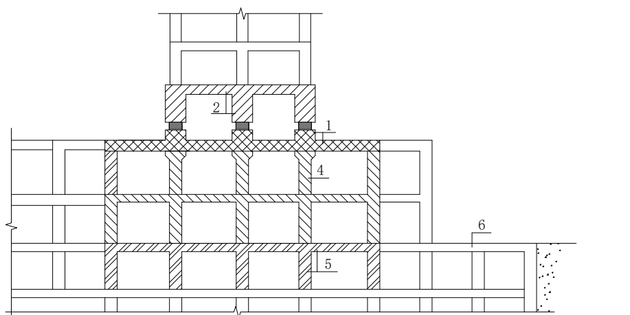
(c) 带大底盘裙房隔震建筑
